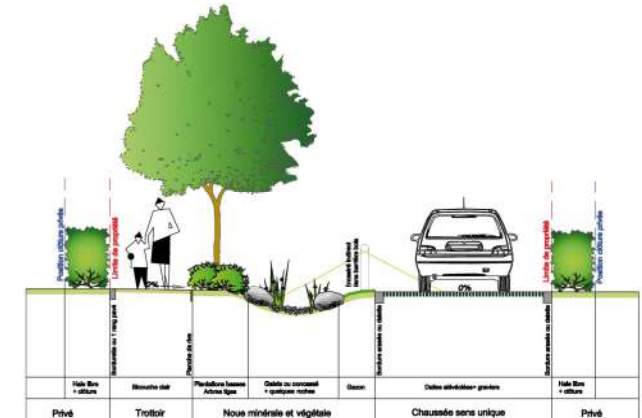
Exemple de traitement de voie en sens unique ou alterné
